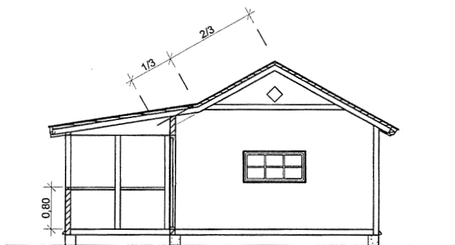
TVERRSNITT
