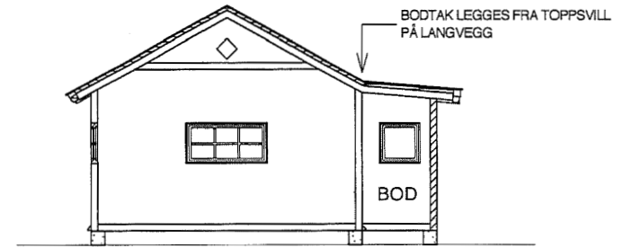
TVERRSNITT, BOD ALT. B PÅ LANGVEGG
