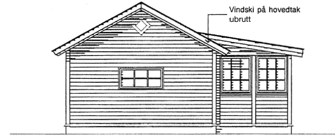
GAVLFASADE
