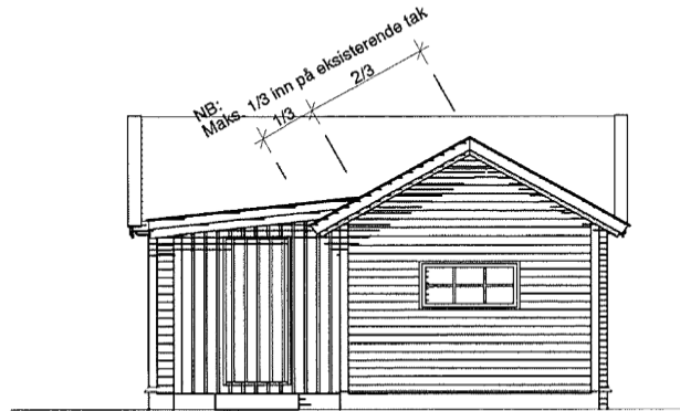
FASADE SOVEROM MED BOD, ALT: A
