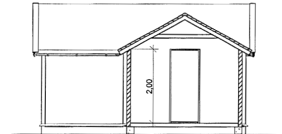
TVERRSNITT, SOVEROM
