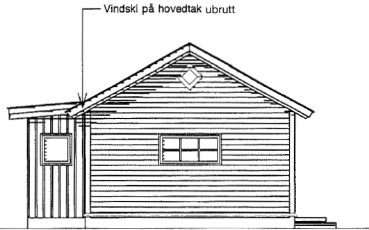
GAVLFASEDE MED BOD, ALT. B
