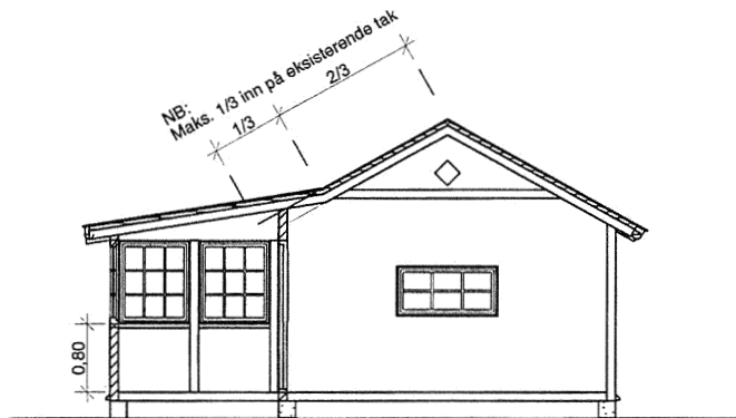
TVERRSNITT
