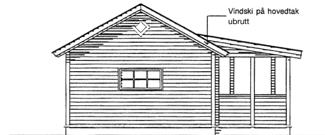
GAVLFASADE
