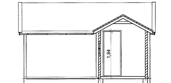
TVERRSNITT, SOVEROM
