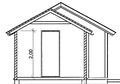
TVERRRSNIITT, SOVEROM
