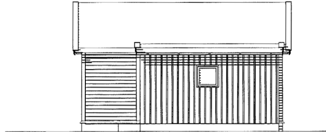
FASADE LANGVEGG MED BOD, ALT: B
