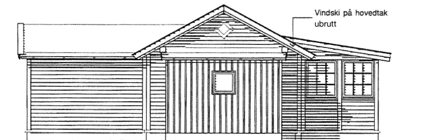
GAVLFASADE (INNGLASSET VERANDA, BOD ALT. B OG SOVEROM ALT. 3)
